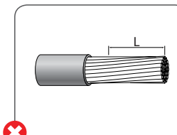
Избыточно снятая изоляция
